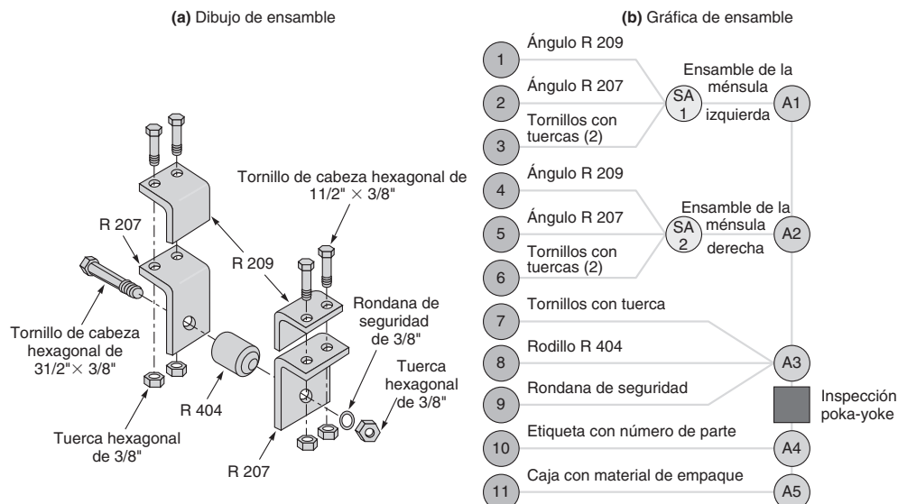
◀ Figura 5.11 Dibujo de ensamble y gráfica de ensamble
