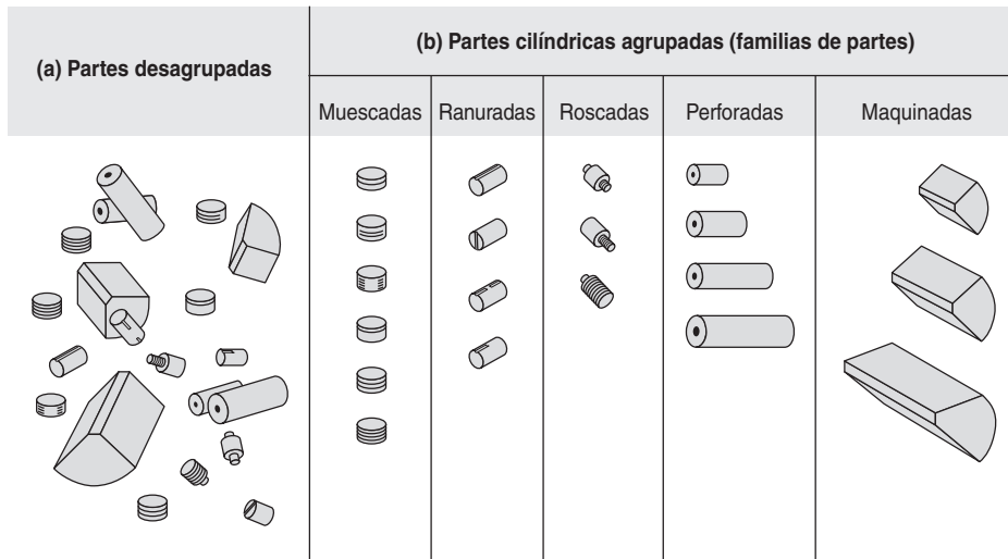
◀ Figura 5.10 Una variedad de esquemas de codificación para tecnología de grupos permite que componentes manufacturados pasen de ser (a) desagrupados a (b) agrupados (familias de partes)
